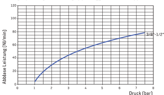
DIAGRAMM DER BETRIEB DES SCHNELLENTLÜFTER BESSER
