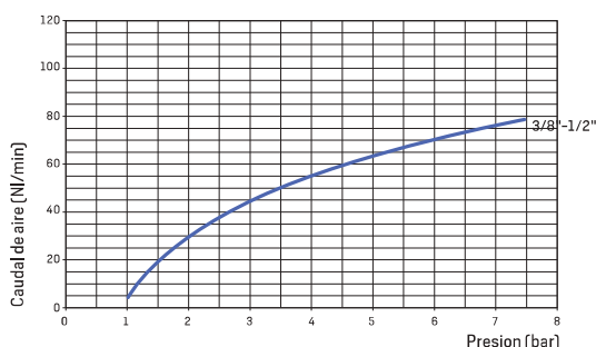
CURVA DE FUNCIONAMIENTO PURGADOR BESSER
